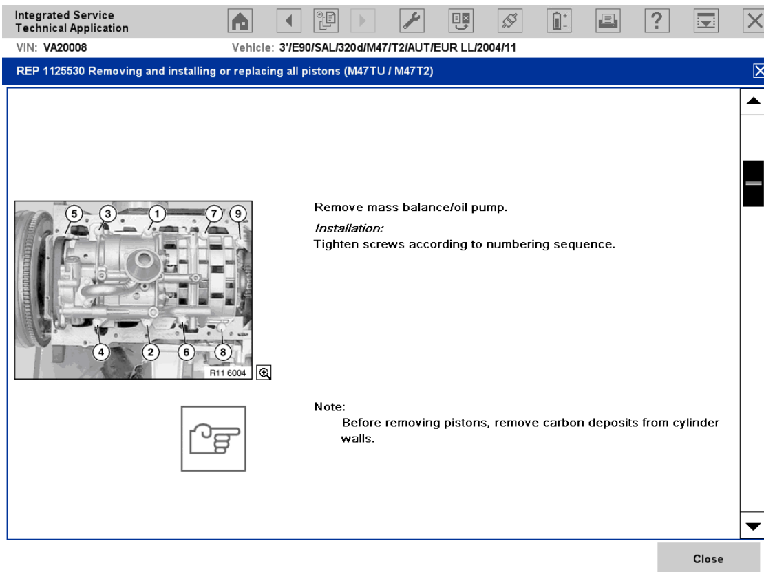
Fig. 3.46 Text document
