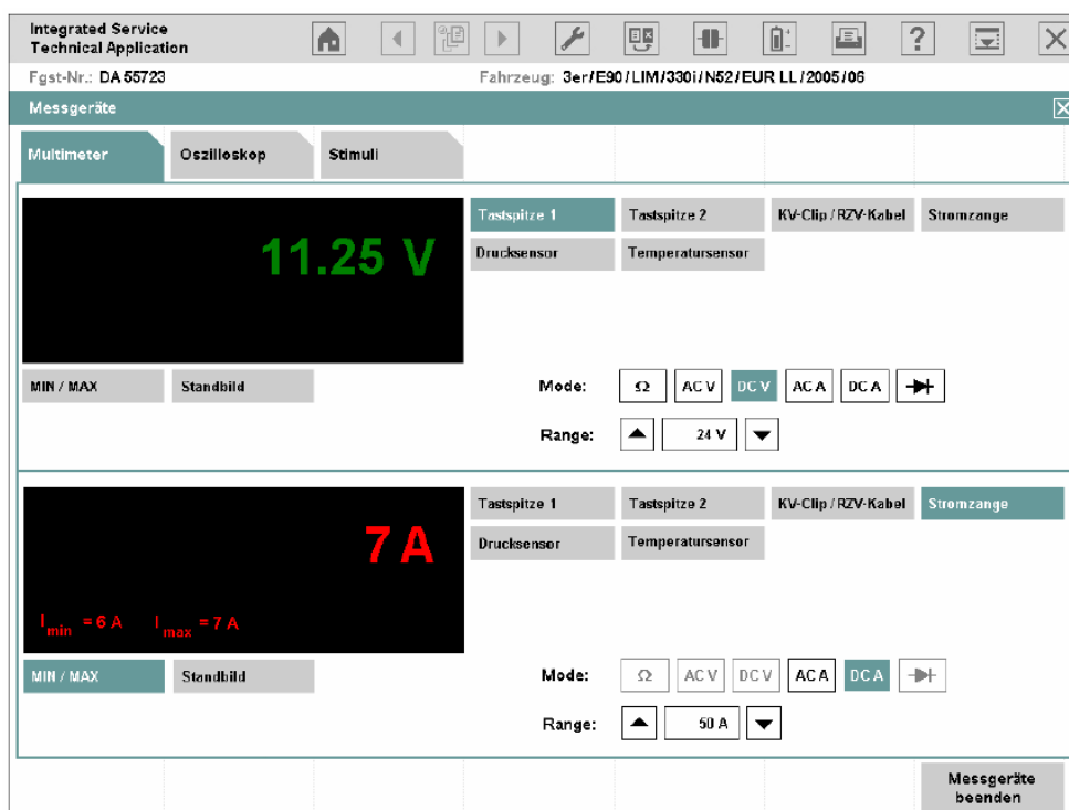
Fig. 3.36 "Multimeter" mask
